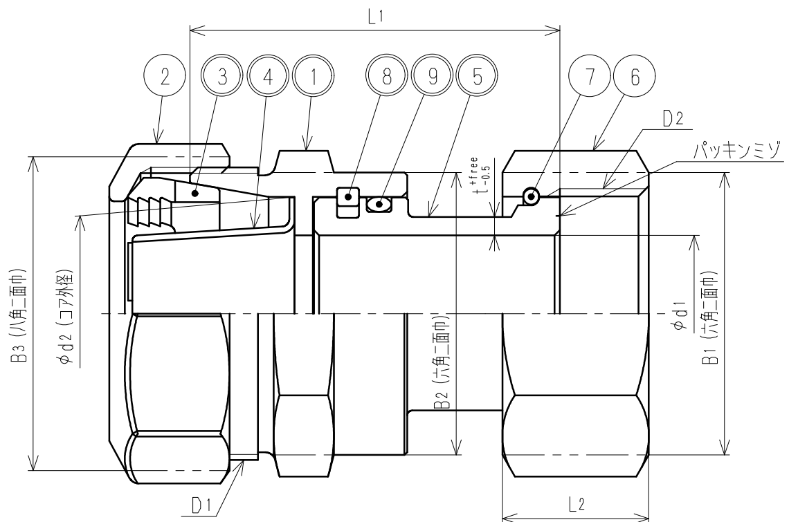
寸法表
